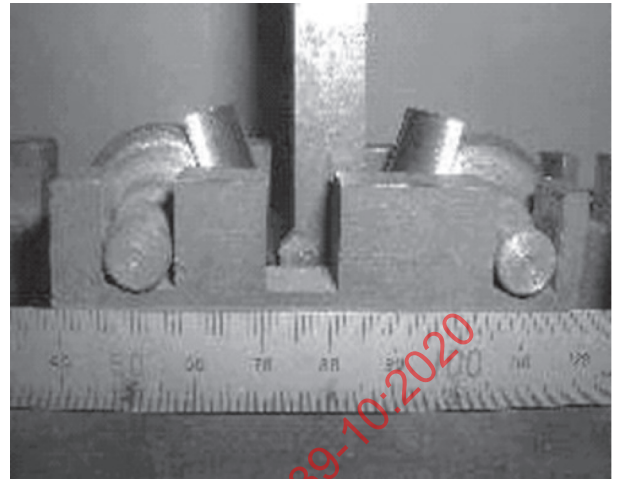
b) Reverse U-bending
