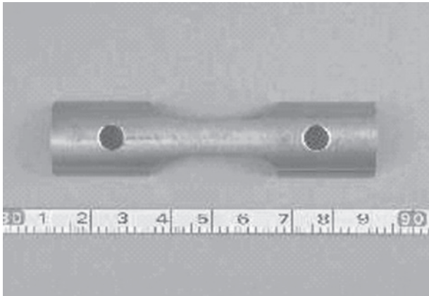
a) Tensile type specimen
