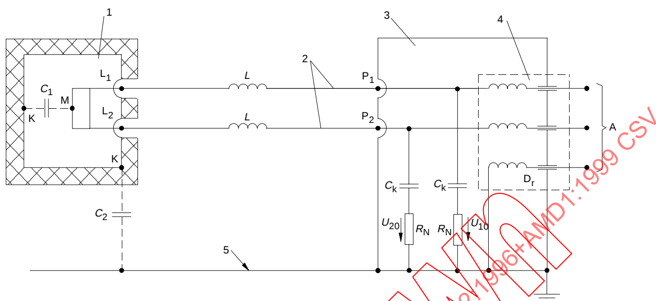
Figure 7a – Schéma du circuit d'alimentation et de mesure
