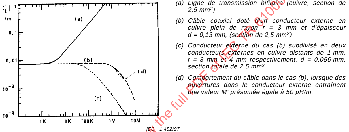
Figure B.2 – Comportement de Z'_t en fonction de la fréquence, pour les configurations de câbles coaxiaux (a), (b), (c) et (d)
