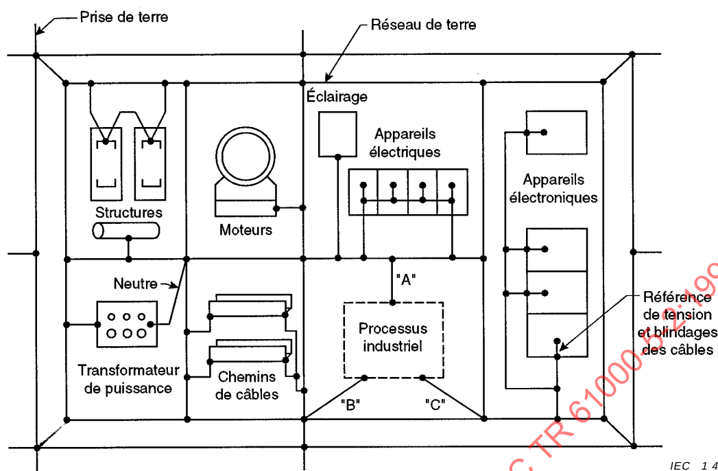
Figure 8 – Principes généraux de connexion des parties conductrices de différents appareils ou systèmes au réseau de terre
