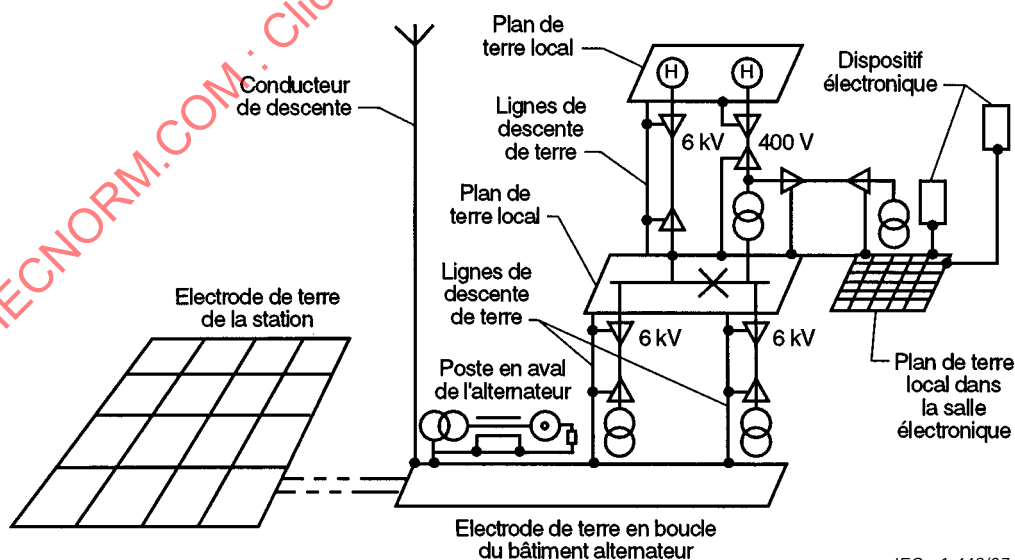
Figure A.4 – Système de terre d'un réseau électrique comprenant des dispositifs électroniques de commande et de surveillance
