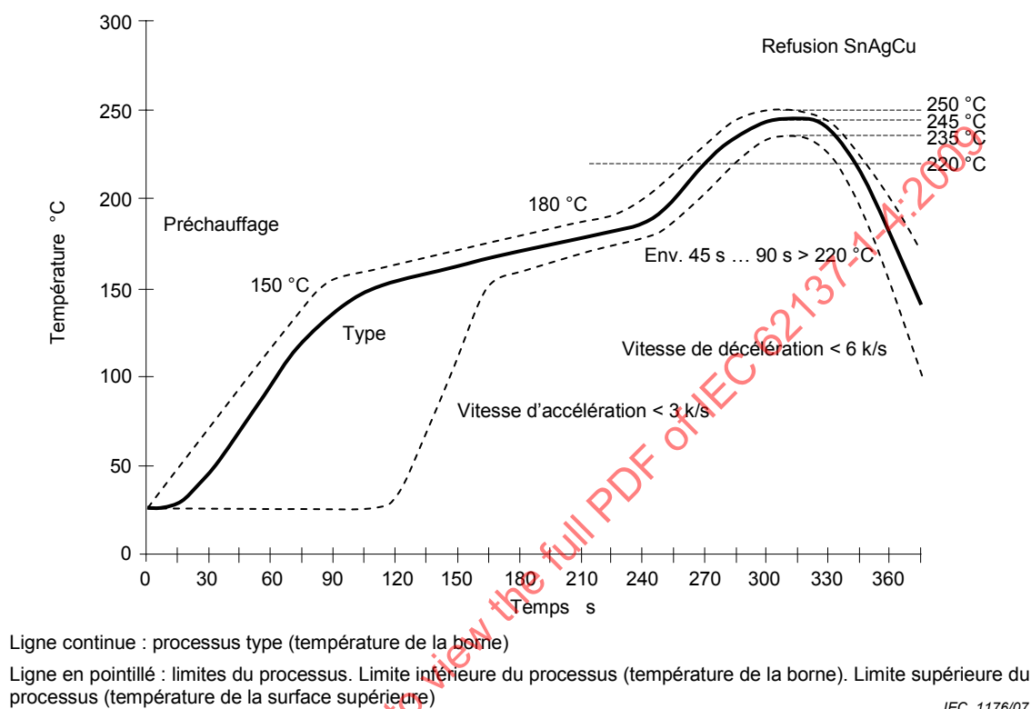
Figure 2 – Profil typique de brasage par fusion
