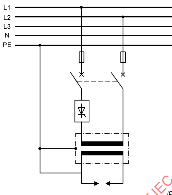
Figure 4 – Exemple de conducteur de protection connecté directement au circuit de soudage (matériel de soudage monopoint, courant alternatif)
