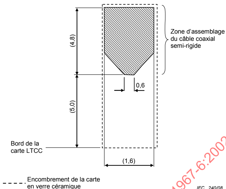
Figure E.7 – Couche 5 (motif de mise à la masse) de la sonde magnétique améliorée
