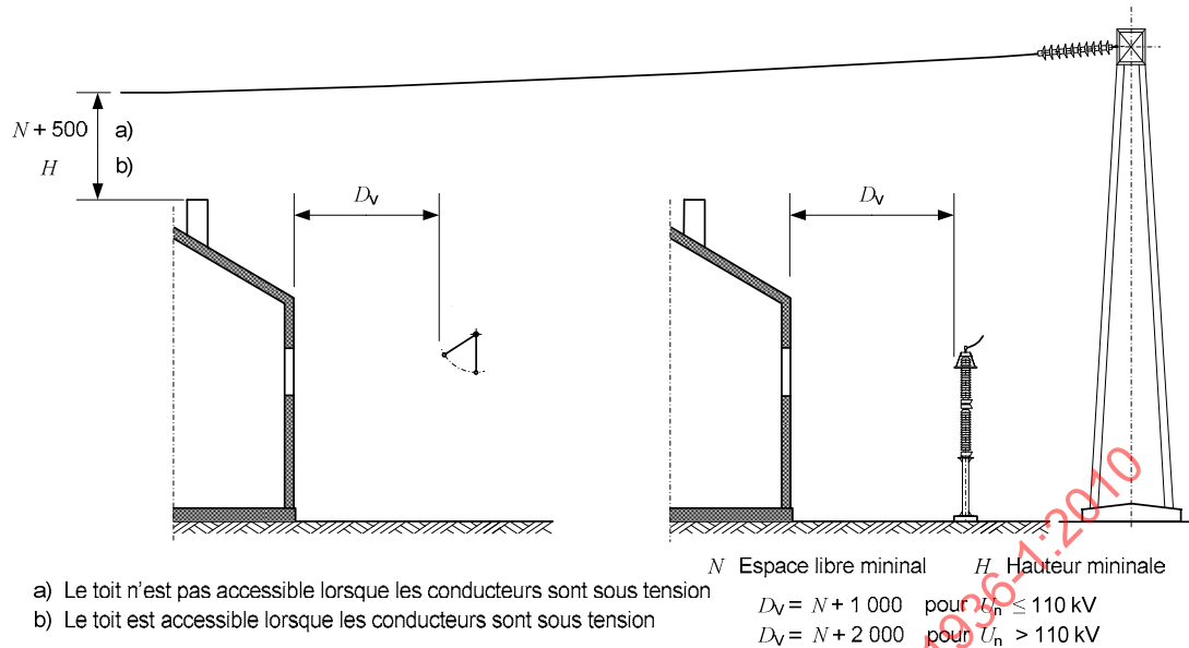
Figure 4a – Mur extérieur avec fenêtres non grillagées
