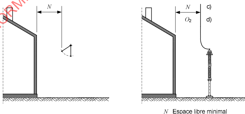
Figure 4c – Mur extérieur sans fenêtre
