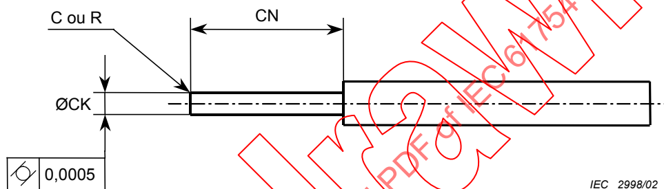
Figure 1b – Broche calibrée pour manchon d'alignement élastique
