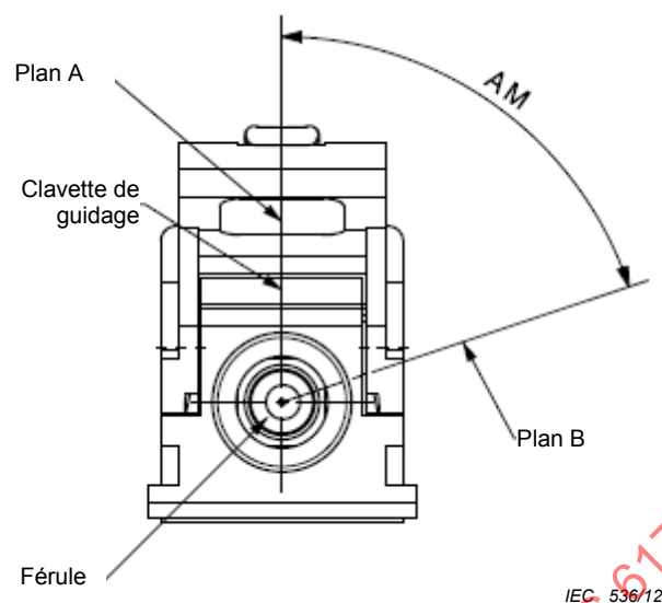
Figure 5 – Interface de connecteur mâle APC simple
