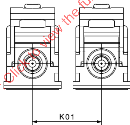
Figure 6 – Interface de fiches duplex
