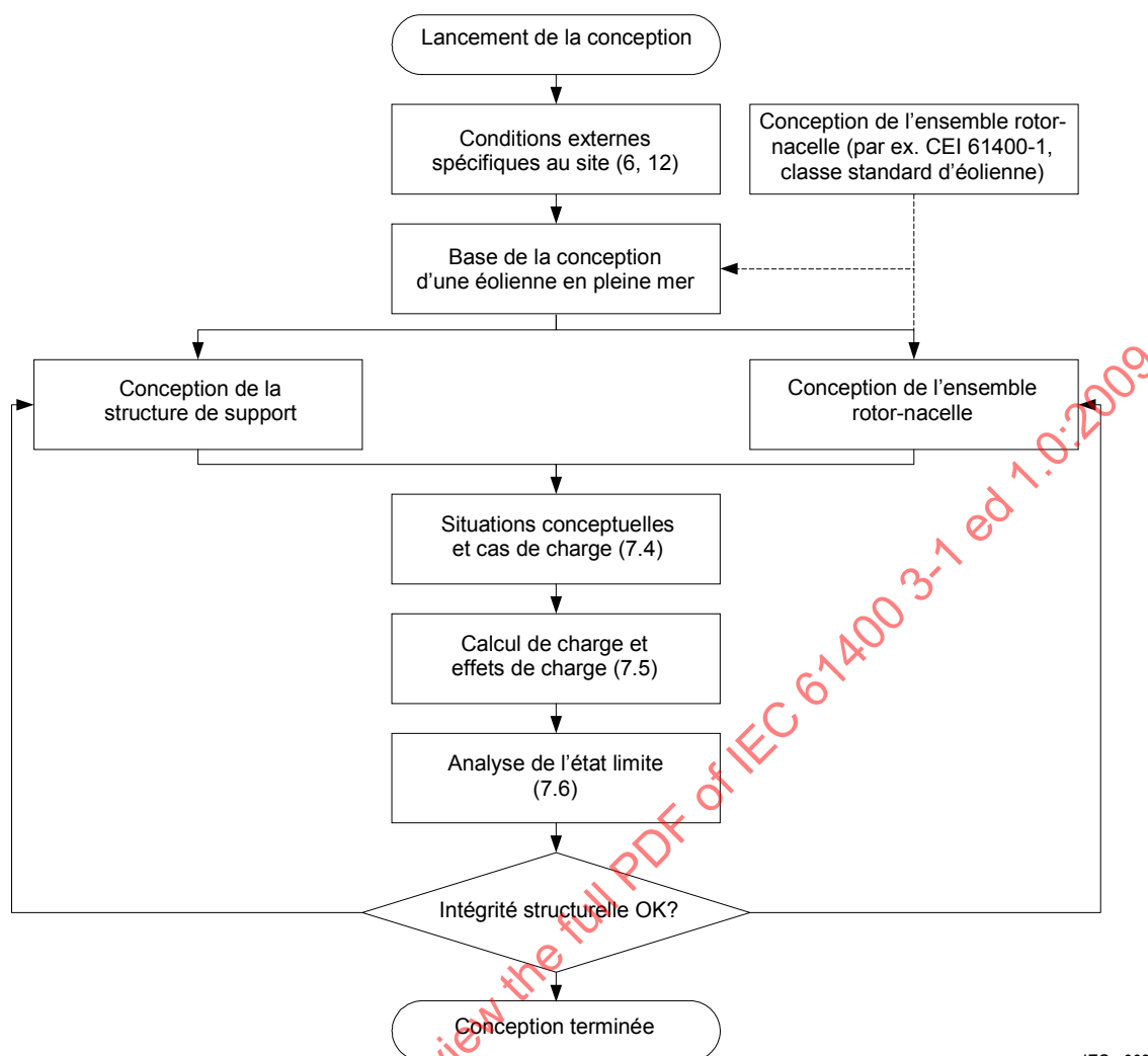
Figure 2 – Processus de conception d'une éolienne en pleine mer
