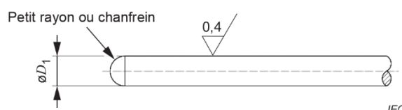
Figure 5 – Calibre pour un contact central femelle
