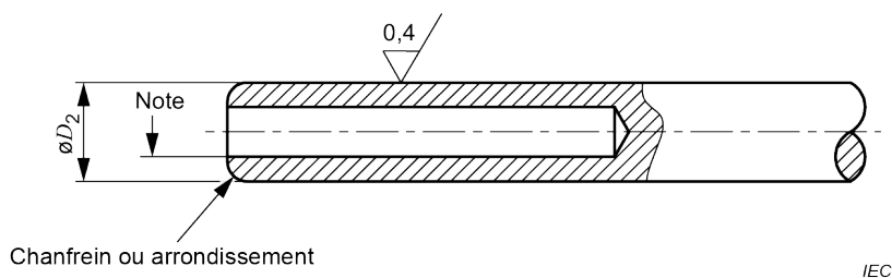
Figure 6 – Calibre pour un contact intermédiaire femelle
