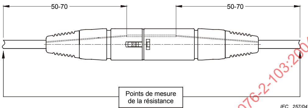
Figure 24 – Accouplement des fiches
