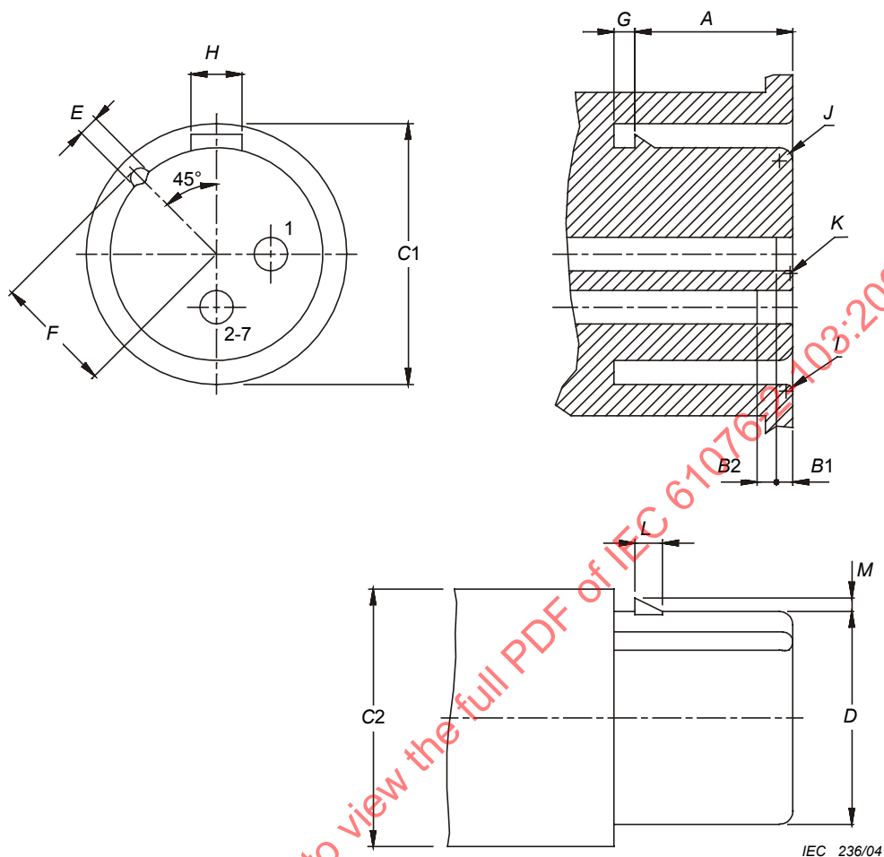
Figure 3 – Connecteur femelle
