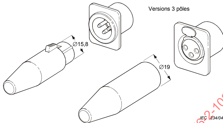
Figure 1 – Caractéristiques communes
