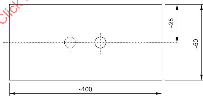
Figure 2 – Taille des éprouvettes d'essai et disposition des électrodes pour l'essai de rigidité diélectrique le long des lignes de colle (rigidité diélectrique sur l'arête)
