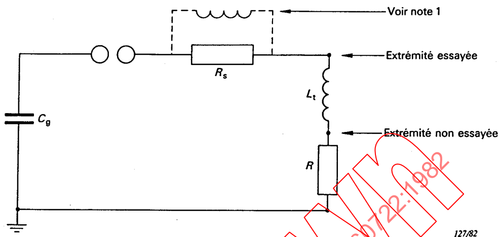
FIG. 8. — Mise à la terre à travers une résistance d'enroulements à basse impédance.
