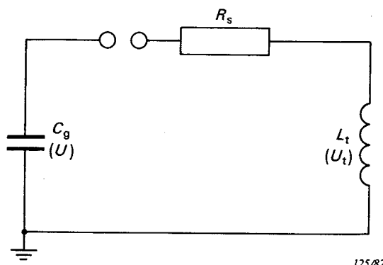
FIG. 6. — Réglage de la queue de l'onde pour les enroulements à basse impédance.
