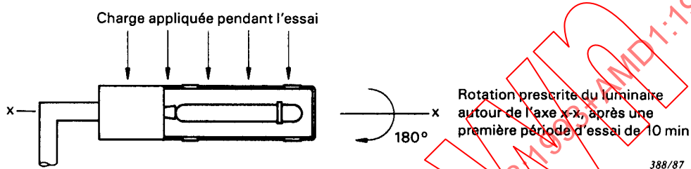
Détail b) – Position d'essai initiale
