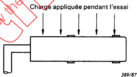
Détail c) – Position lors de la répétition de l'essai
