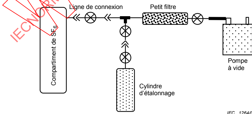
Figure B.1 – Montage d'échantillonnage du gaz SF 6 : évacuation
