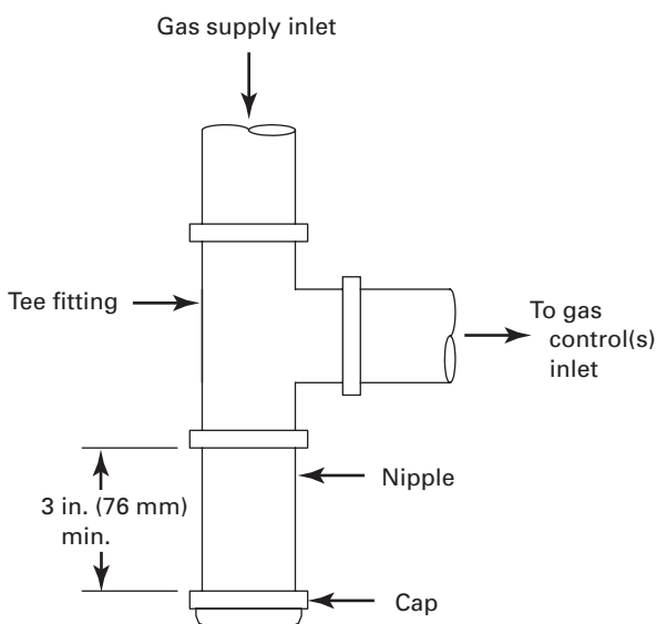
Fig. 1 Sediment Trap
